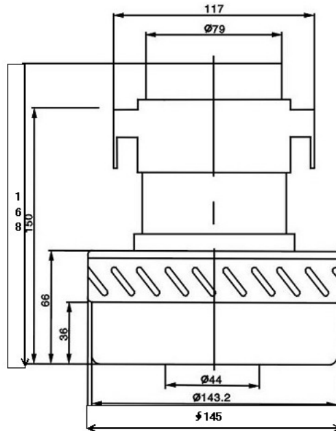
PX-PR-LG Technical Parameters
